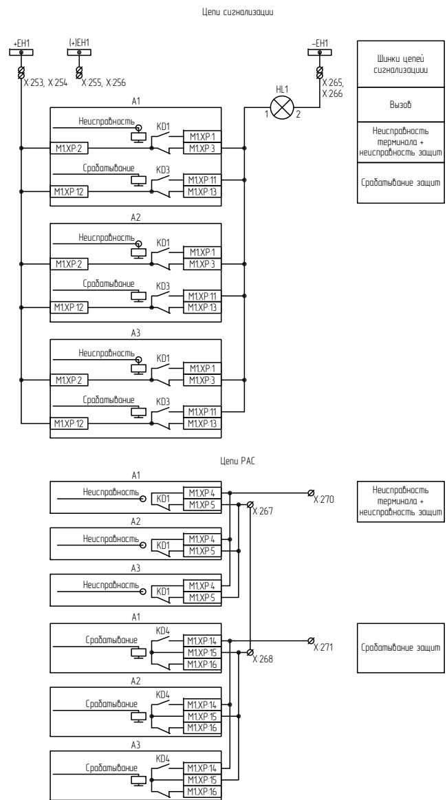
Рисунок В.8 – Схема электрическая принципиальная (часть 8)
