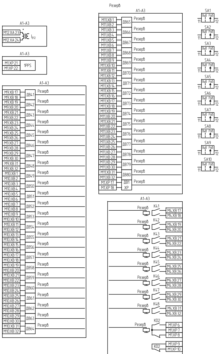
Рисунок В.9 – Схема электрическая принципиальная (часть 9)
