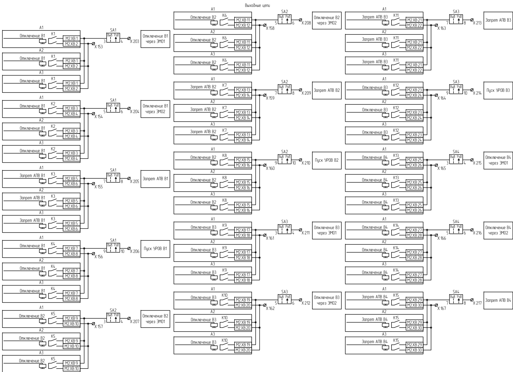
Рисунок В.5 – Схема электрическая принципиальная (часть 5)
